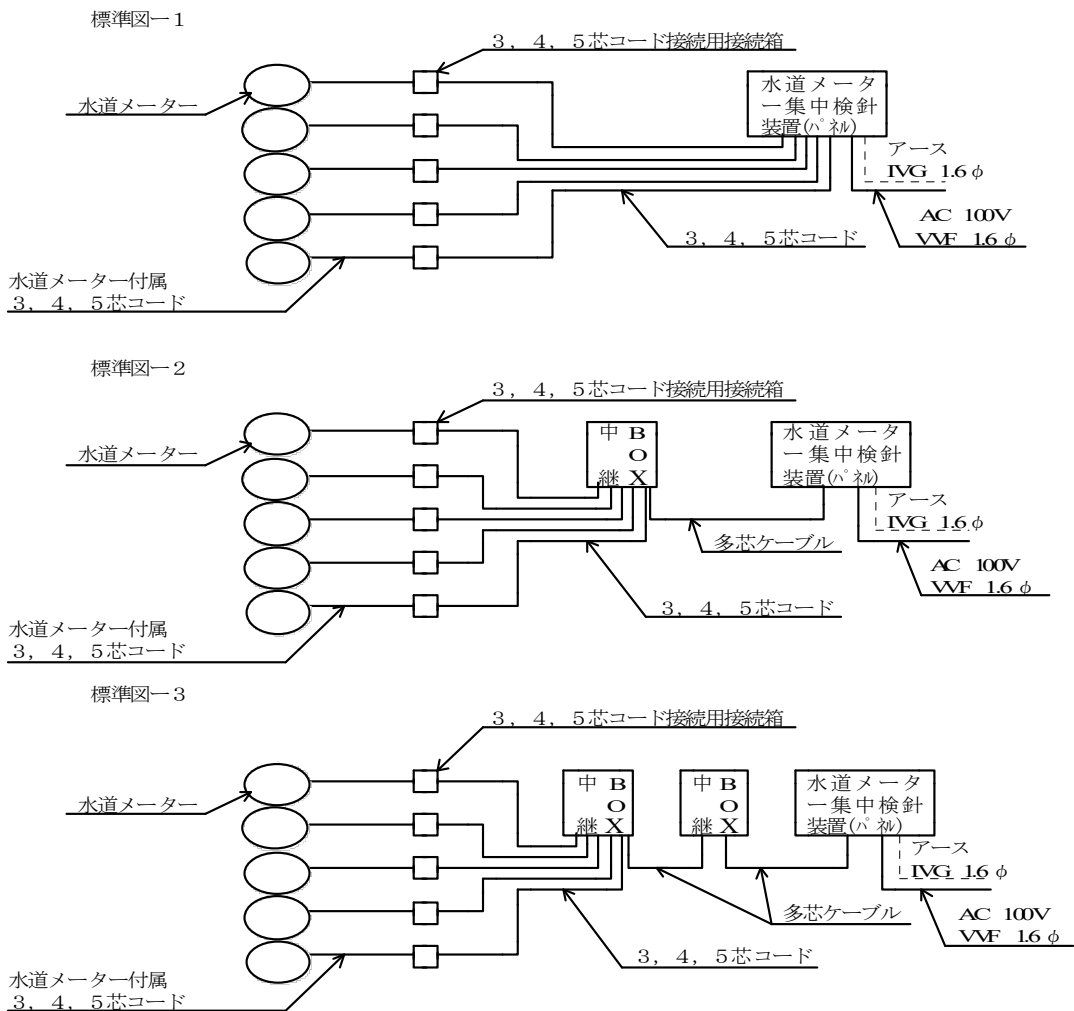
集中検針装置標準図
