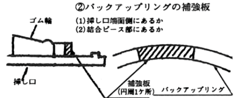
②バックアップリングの補強板
