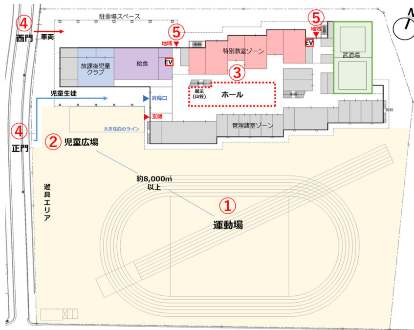
1階平面図兼配置図イメージ※上記番号に対応
