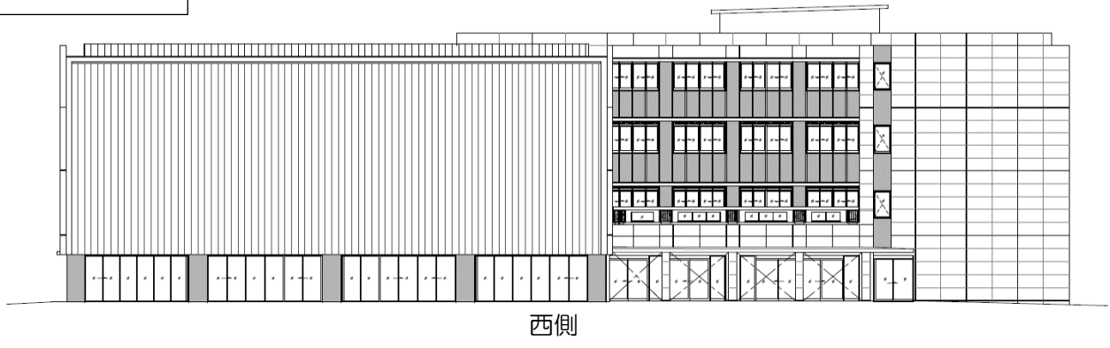
校舎棟立面図
